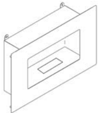
modello da incasso a parete (misure incasso: base 70cm h. 50 cm profondità 23 cm.)
