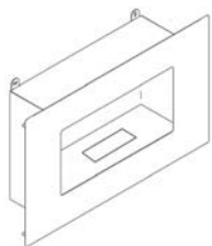
modello da incasso o parete (misure incasso: base 70cm h. 50 cm profondità 23 cm.)
