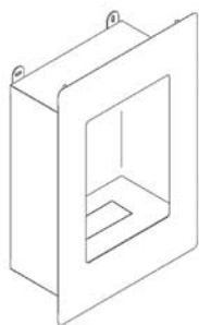
modello da incasso o parete (misure incasso: base 40cm h. 58 cm profondità 23 cm.)
